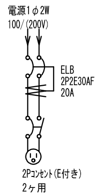
結線図
